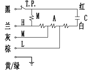
接线图:
